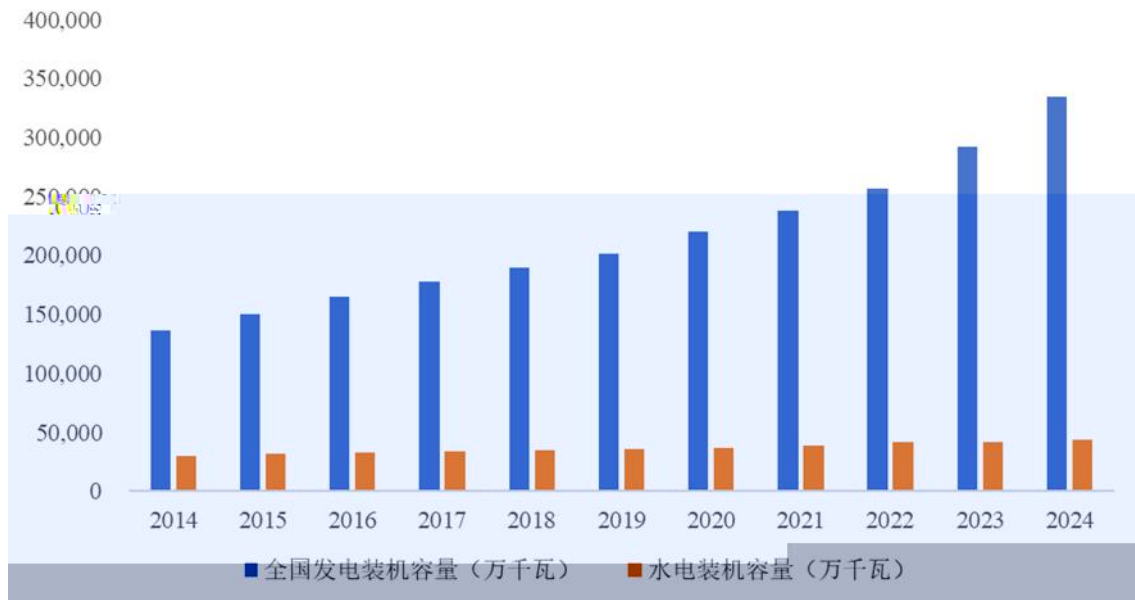
2014年至2024年全国发电装机容量
